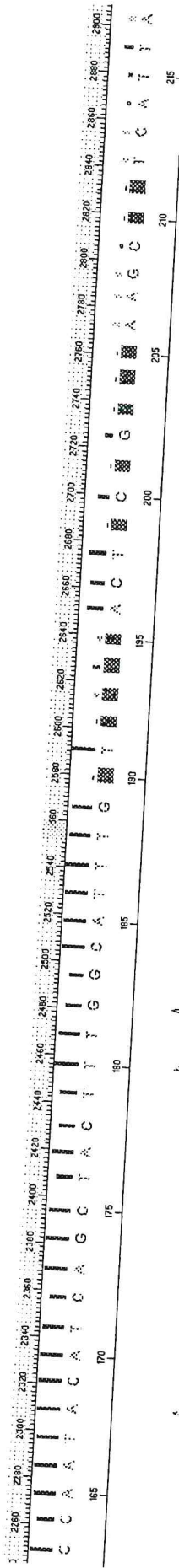
Elettrogramma di sequenziamento con metodica Sanger
